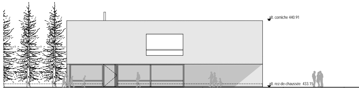
FACADE NORD / EST
